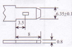
Optional Terminal F2 (Fasten Tab No.250A)
